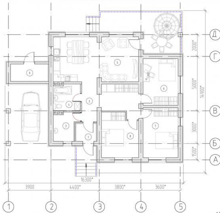
План на отм.0,000 (тип 1-100м²)
