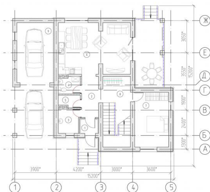
План на отм.0,000 (тип 2-150м²)
