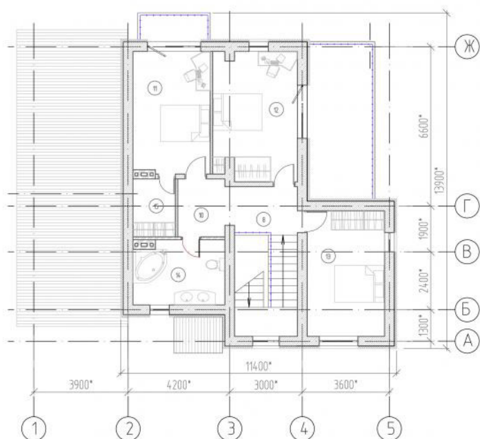
План на отм.+3,300* (тип 2-150м²)
