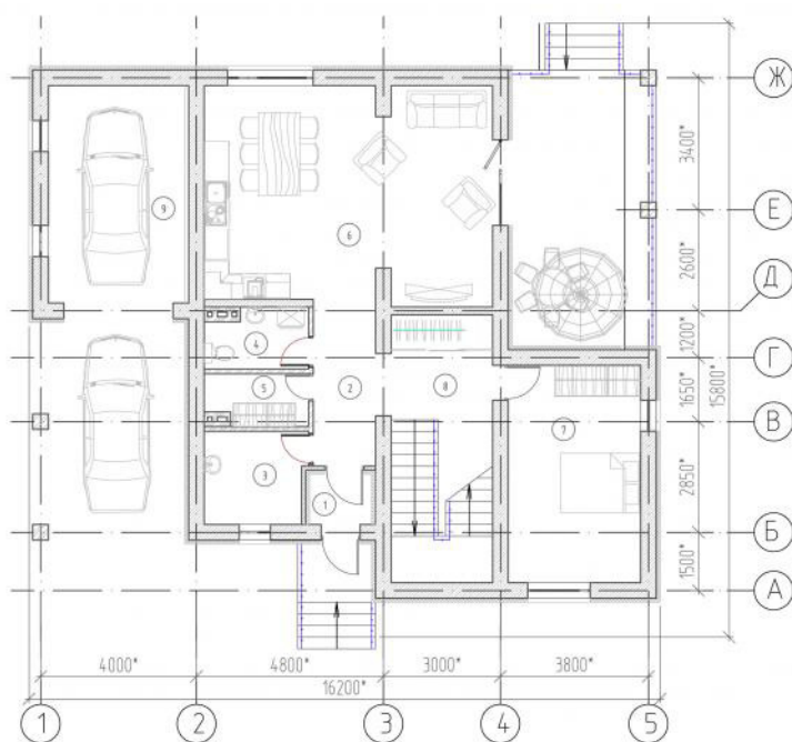
План на отм.0,000 (тип 3-200м 2 )
