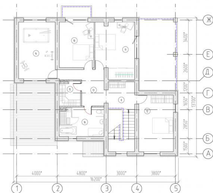
План на отм.+3,300* (тип 3-200м²)
